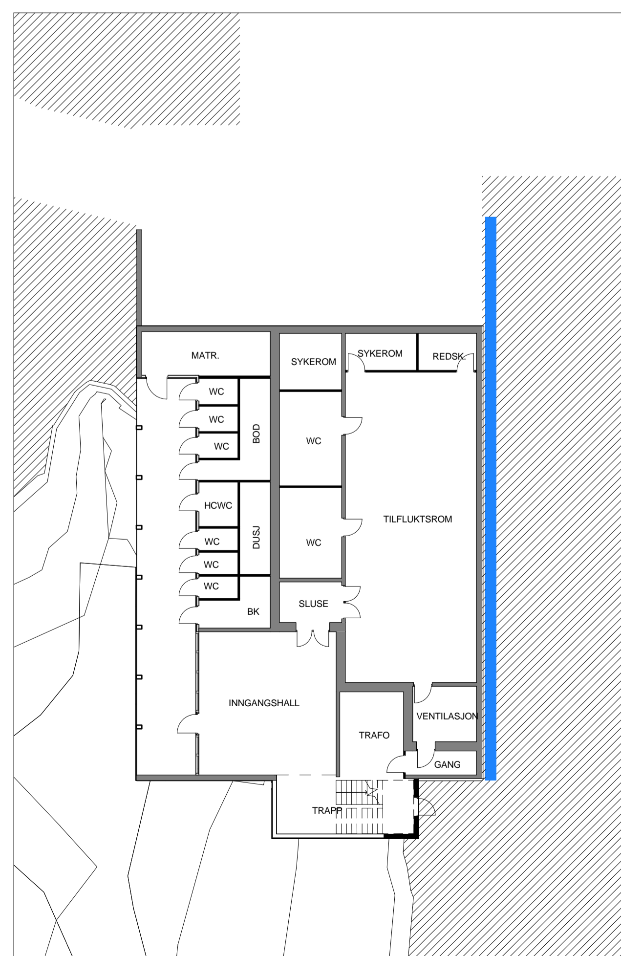
Utbetringar drenering Uetg - hovedbygg
