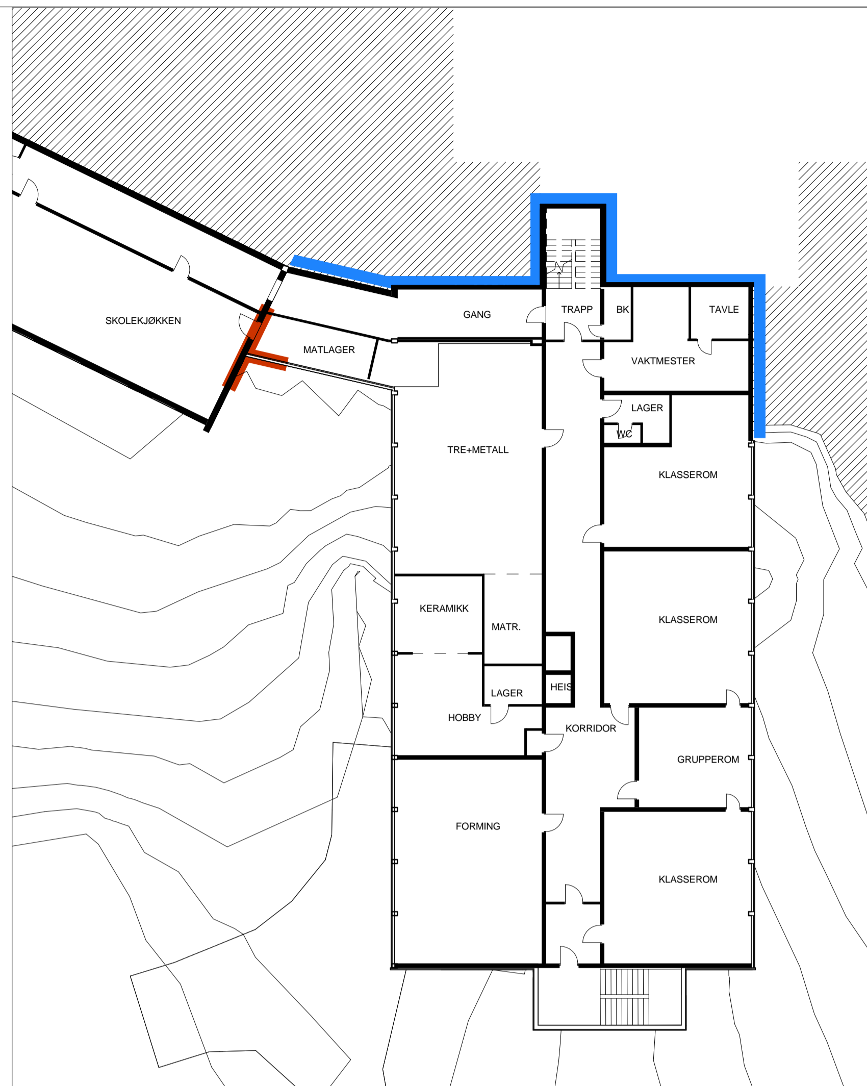
Utbetringar vannskader / drenering 1etg
